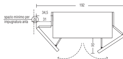
pianta - ingombri
